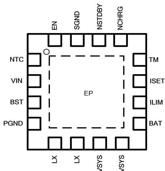
图 3. SLM6807 引脚封装图
